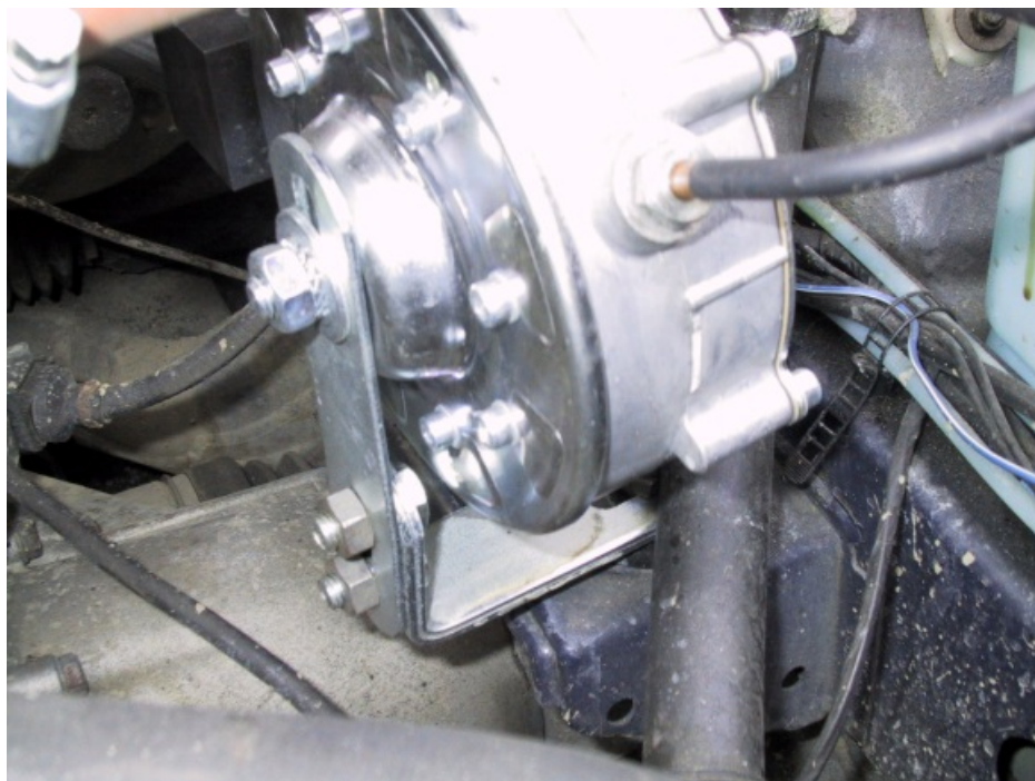
Obrázek 3b, umístění regulátoru tlaku - detail
