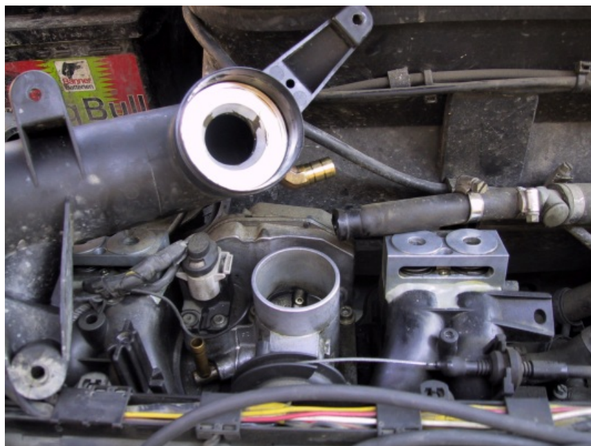
Obrázek 1b, umístění směšovače detailní provedení
