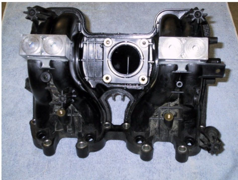
Obrázek 1c, upravené sání
