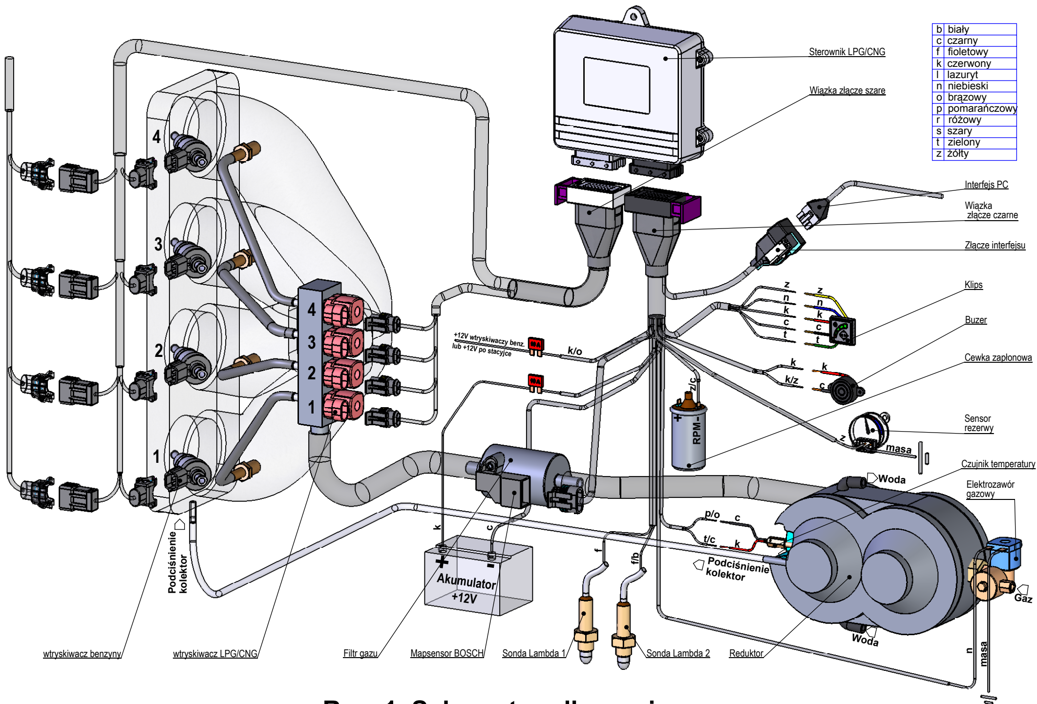
Rys. 1 Schemat podłączenia
