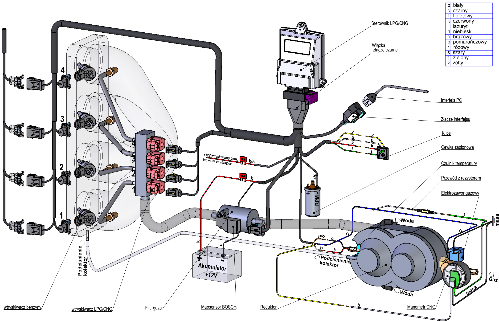
Rys. 1 Schemat podłączenia
