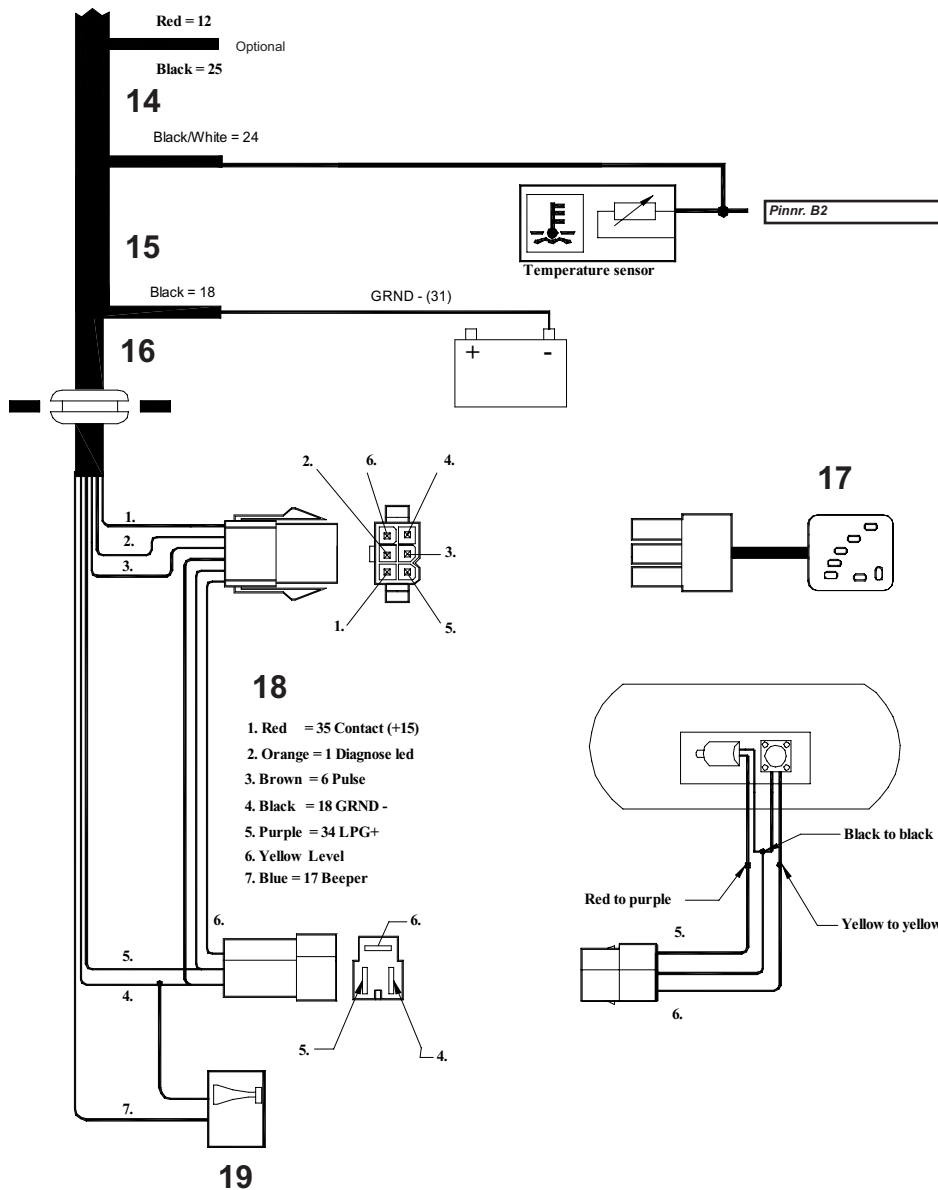
Position of connection / Plaats aansluiting Position connection / Sitio empalme
