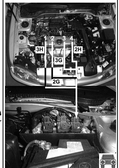
Position of interruption / Plaats van onderbreking / Position du déconnection
