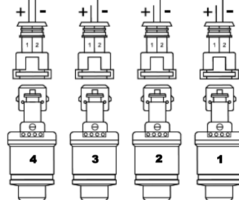
WTRYSKIWACZ BENZYNY
